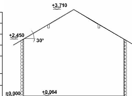
ŘEZ
