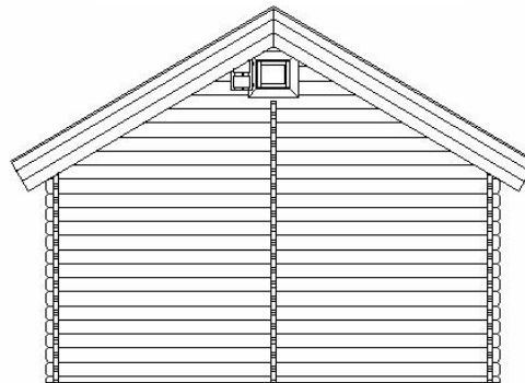
ZADNÍ POHLED
